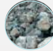
Clinoptilolite
